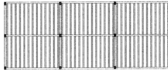
Planta de vigotas pré-moldadas
